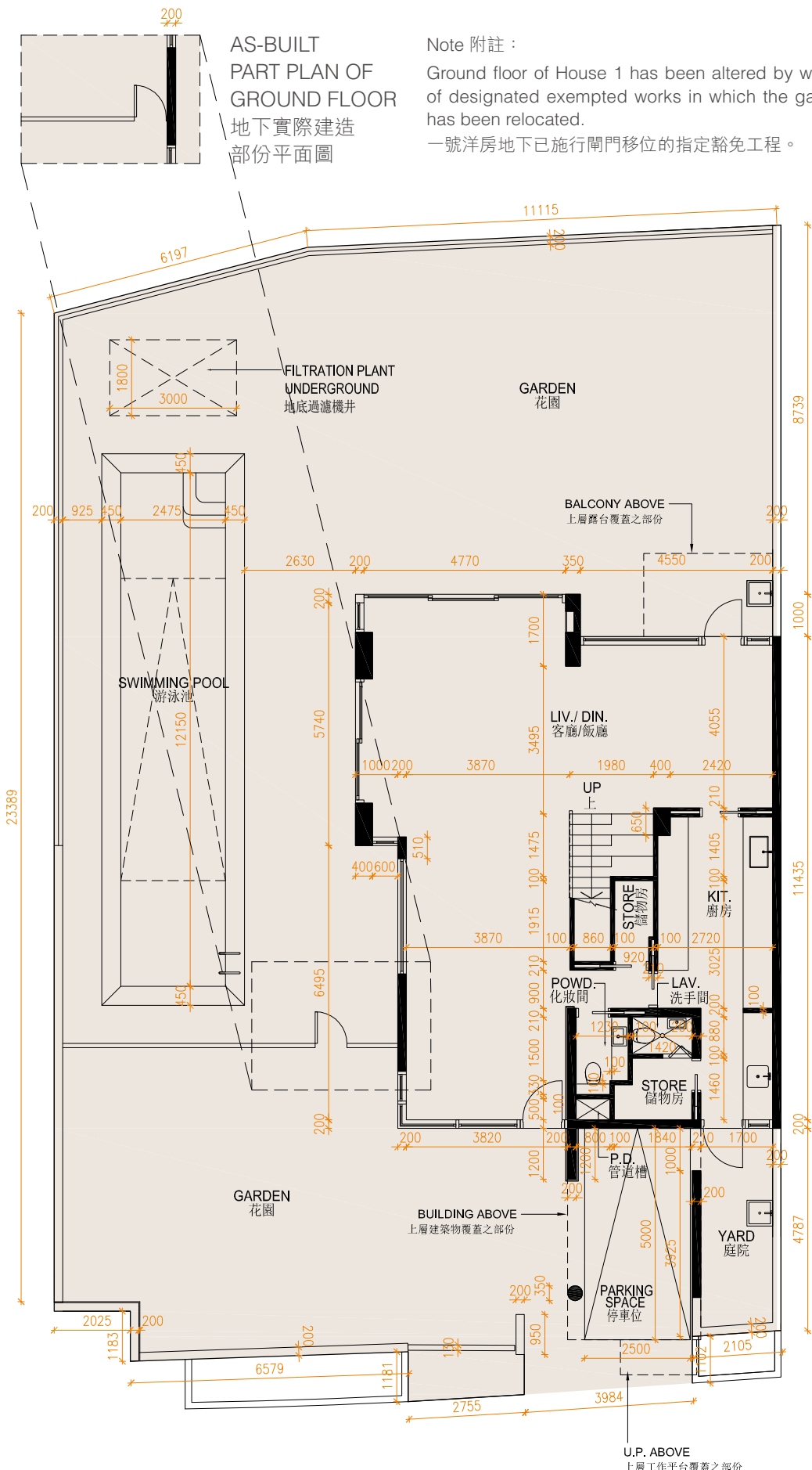
GROUND FLOOR PLAN 地下平面圖
