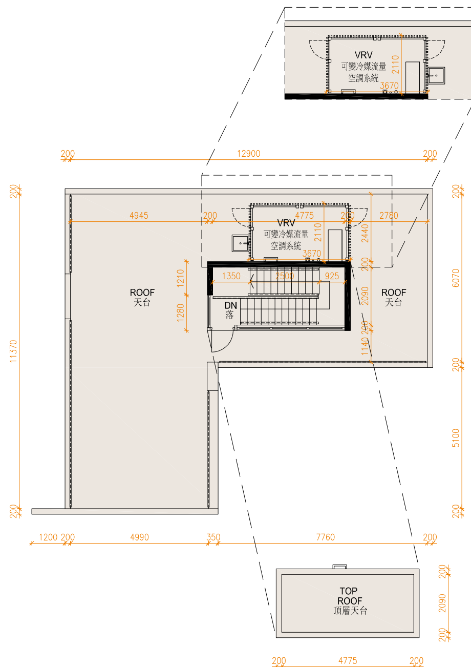
TOP ROOF PLAN 頂層天台平面圖
