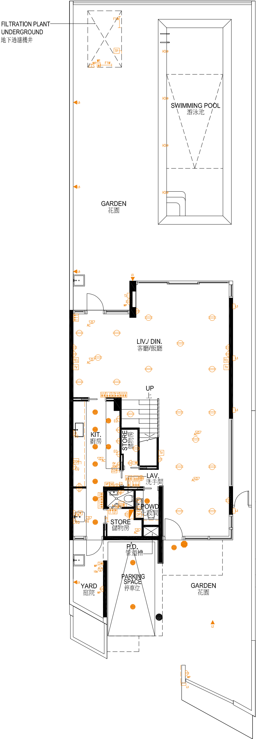
GROUND FLOOR PLAN 地下平面圖
