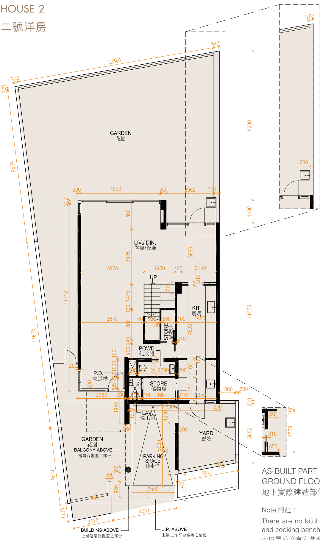
GROUND FLOOR PLAN 地下平面圖
